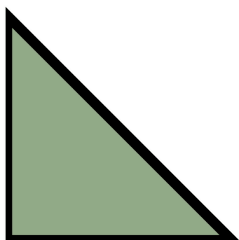
RETTVINKLET TREKANT
