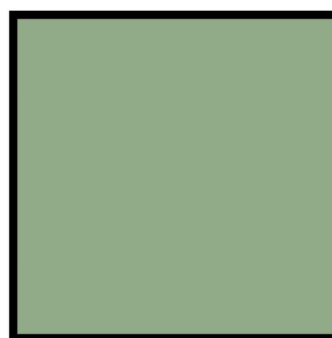
KVADRAT
